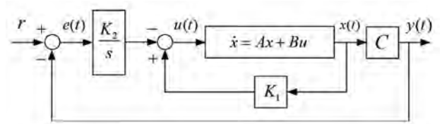
Fig.4 最適ロバストサーボシステム
