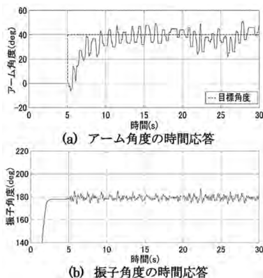
Fig.6 アームと振子角度の時間応答
