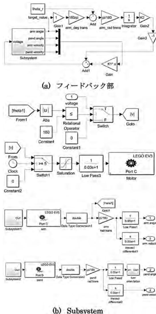
Fig.5 simulinkのブロック線図
