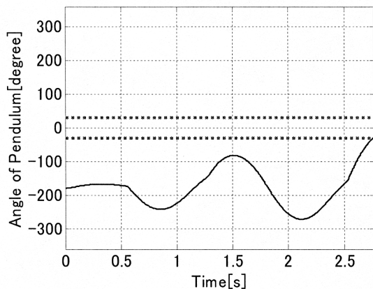
図9 振り角度 \alpha の時間応答
