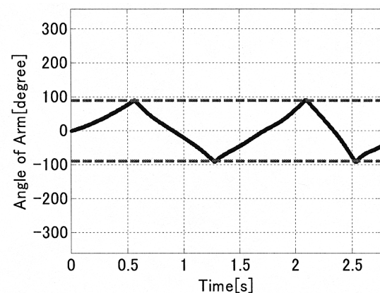
図8 アーム角度 \theta の時間応答
