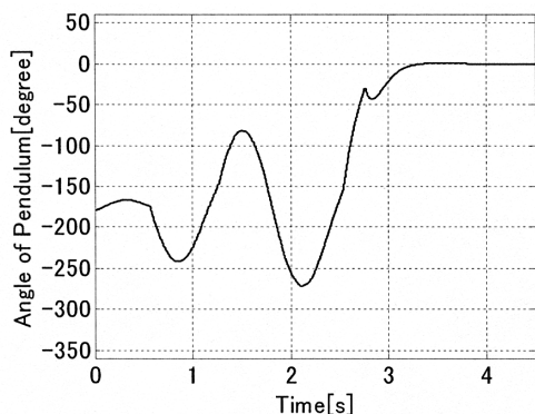
図10 振り角度 \alpha の時間応答
