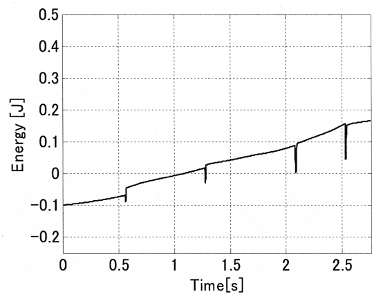
図7 \dot{E} の時間応答
