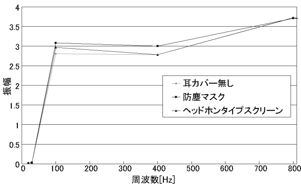
図17：通常の音波を録音した時の耳カバーの有る場合と無い場合での振幅の差異
