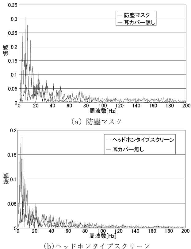
図：19 野外での耳カバーによる風音の低減
