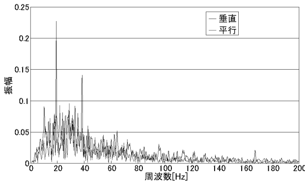
図8：マイクを耳型に挿入して風音を録音したときにマイクの向きを垂直にした場合と平行にした場合のスペクトラムの差異（風量：強）
