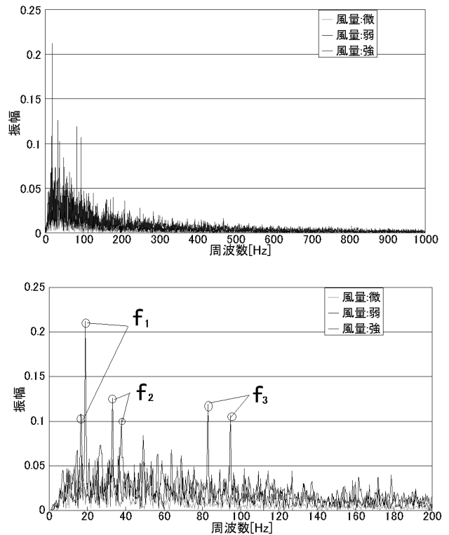
図4：風量設定の違いによるスペクトラムの差異 (向き：垂直)
