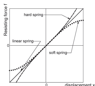
図2 非線形ばね特性
