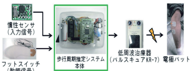
Fig. 10 遊脚期推定システムの装着
