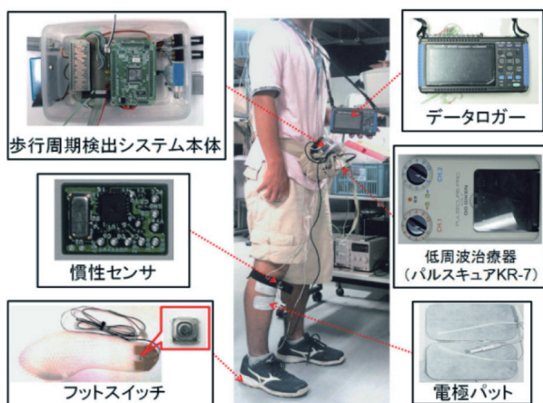
Fig. 1 遊脚期検出システムの装着
