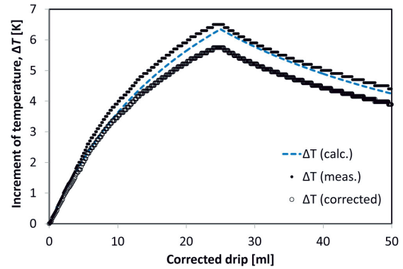
図7 補正した温度曲線。温度の各データを、中和反応に関わったイオンの物質質量と溶液の容積とから、中和熱を補正する方法とした。
