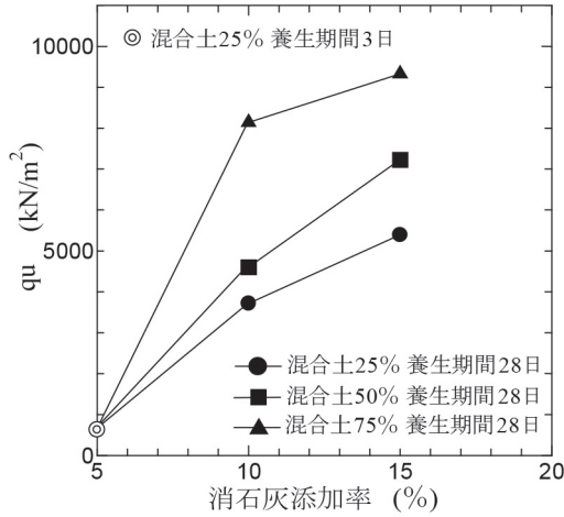
図-3 qu ~消石灰添加率
