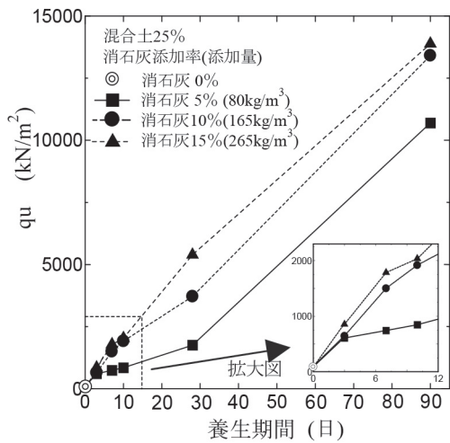
図-4 qu ~養生期間関係
