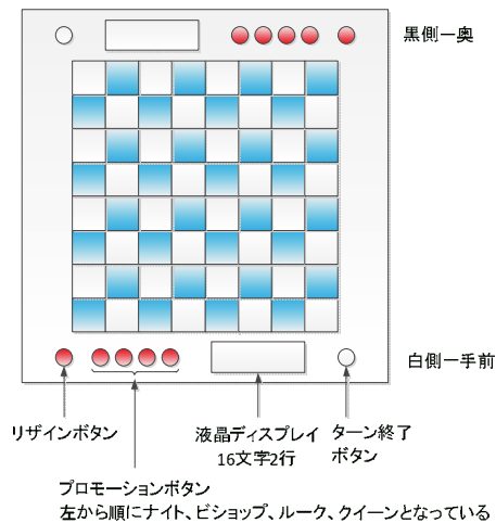
図 2.2 チェスボードの外部の構成
