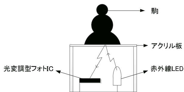
図 1.2 フォトリフレクタの動作の様子
