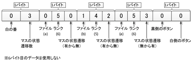
図 3.9 各ビットの 10 進数で表現した通信データ
