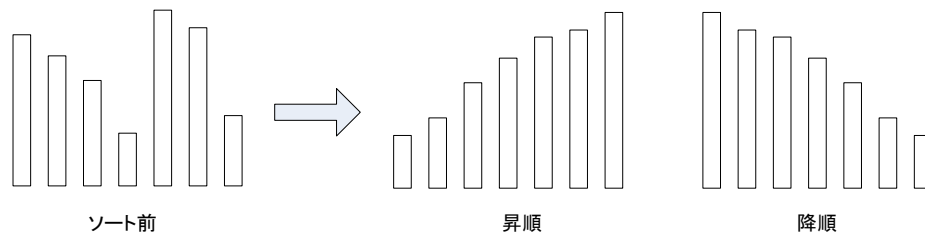
図1 昇順と降順
