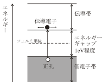
図3 真性半導体のバンド構造
