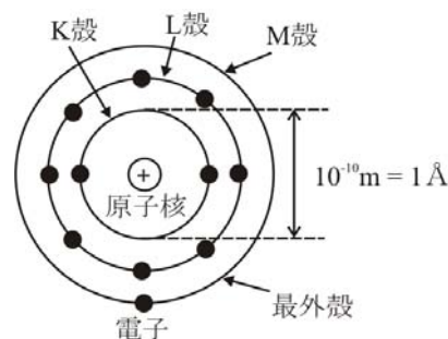
図 1 原子の構造
