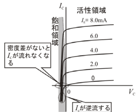
Fig.8 飽和領域
