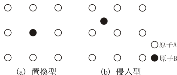
図 3 不純物欠陥
