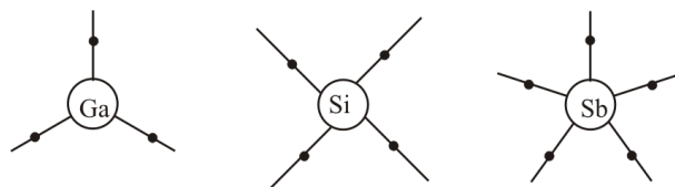
図 2 III族、IV族、V族元素の結合手
