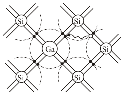
図 5 p 型半導体
