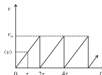
図 2 電界中のドリフト運動
