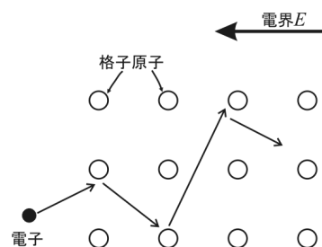
図 1 結晶中の電子の運動
