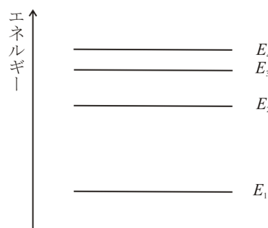
図 1 孤立原子の準位
