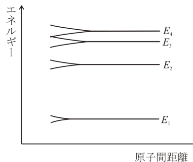
図 2 2 原子の準位
