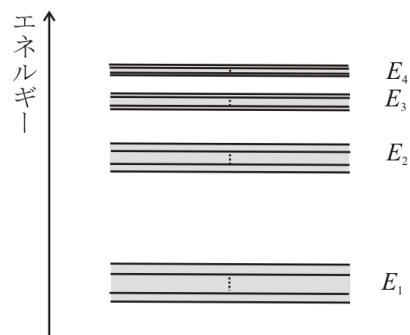
図 3 固体中の準位
