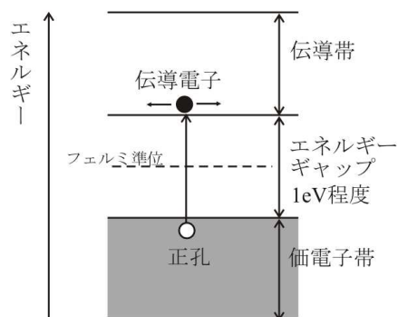
図4 真性半導体のバンド構造
