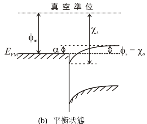
Fig.1 オーム接触
