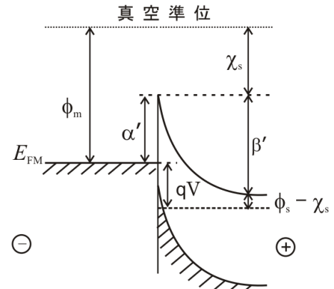
Fig.3 逆方向バイアス
