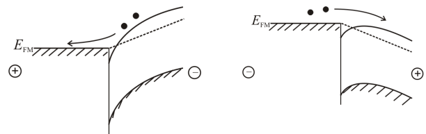
Fig.4 オーム接触(電圧印加時)
